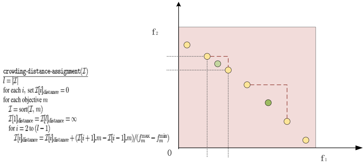
图 28 NAGA-II 算法拥挤距离计算示意图
