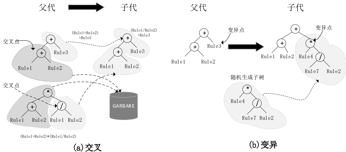
图 18 遗传编程算法架构图
